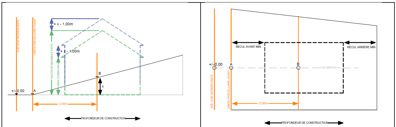
Coupe schématique
