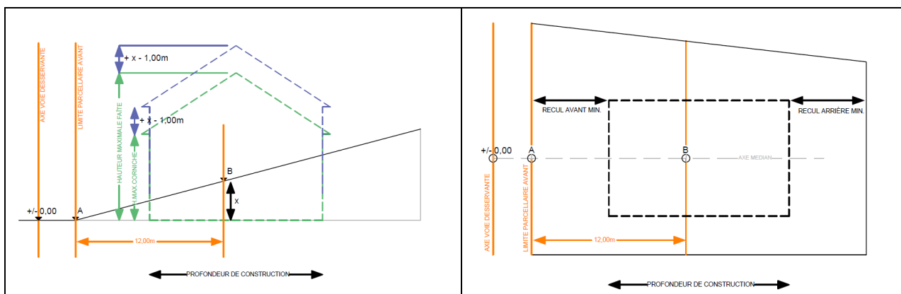
Coupe schématique
